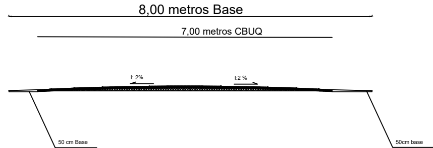
CORTE TRANSVERSAL PISTA DE ROLAMENTO
